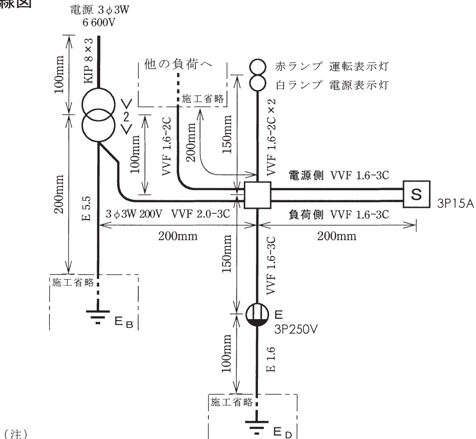
図1. 配線図
